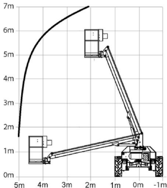
DIAGRAMME TOUR PIVOTANTE CENTRÉE
